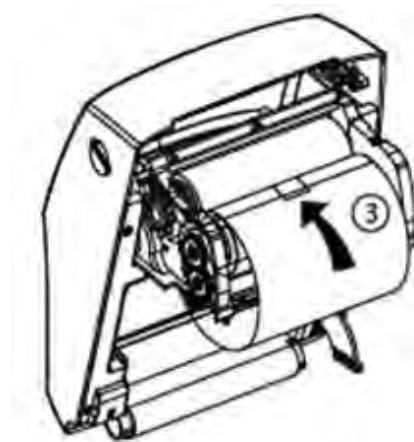
Рисунок 17. Установка ленты
